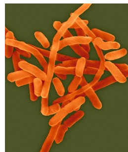
Рис. 9. Вверху: вот так два ядовитых вещества превращаются в одно полезное. Включение формальдегида и фенола в состав аминокислот — блестящий пример биodeградации. Синтез серина из метанола осуществляется некоторыми метилотрофными бактериями (например, Methylobacterium aminofaciens ), тирозина из фенола — Citrobacter freundii . [Рисунок автора]. Внизу слева: метилотрофные бактерии M. capsulatus . Внизу справа: бактерии C. freundii в световом микроскопе. Фотограф Деннис Кункель. [Изображения с сайта https://pixels.com/ ]
