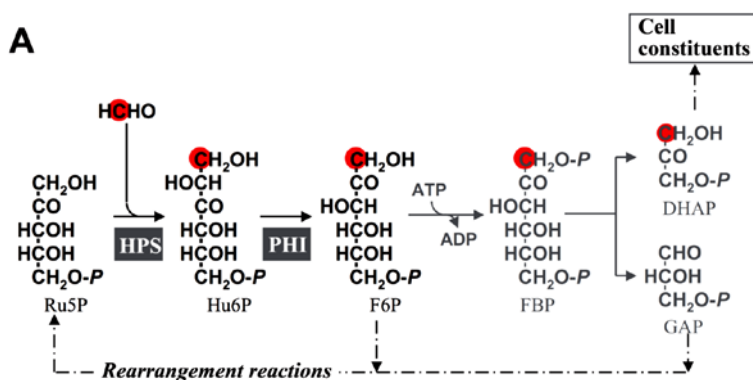
Рис. 7. Один из путей утилизации формальдегида метилотрофными бактериями, по [24], с изменениями. Фактически, это та самая реакция Бутлерова, которая, согласно современным представлениям, привела к появлению сахаров в первичном океане древней Земли, а впоследствии — и жизни на ней
