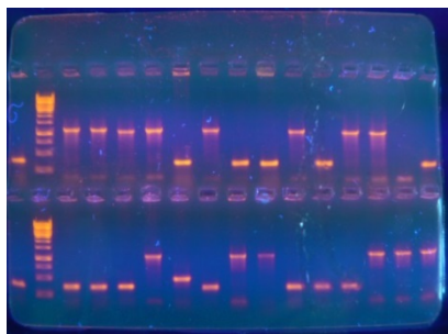
Рис. 7. Слева: электрофореграмма ДНК в полиакриламидном геле после окрашивания флуоресцентным красителем. Справа: акриламид. Изображения с сайта Википедии
