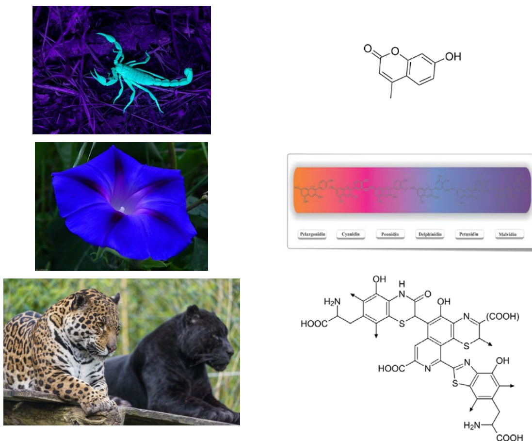
Рис. 12. Слева сверху: этот скорпион, угодивший в луч ультрафиолетовой лампы, флуоресцирует зеленовато-голубым светом, поскольку в его кутикуле содержится метаболиты ароматической природы. Изображение с сайта https://www.alamy.com . Справа сверху: 4-метилумбеллиферон, флуорофор кутикулы скорпиона. Изображение с сайта https://www.ebiochemicals.com . Слева в центре: яркая и контрастная окраска цветов ипомеи обусловлена содержанием в них разнообразных антоцианов. Изображение с сайта Photo.i.ua. Справа в центре: разнообразие структур и окрасок антоцианов. По [28]. Слева внизу: ягуары ( Panthera onca ) разного окраса, обусловленного различным соотношением черного эумеланина и желтовато-коричневого феомеланина в волосах. Изображение с сайта https://w-dog.ru/wallpapers . Справа внизу: химическая структура феомеланина — коричневого пигмента волос млекопитающих. Все эти соединения являются продуктами метаболизма ароматических аминокислот и, в конечном итоге, шикимовой кислоты
