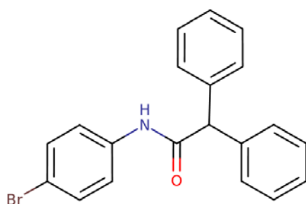
Рис. 1. Слева: пространственная структура N-4'-бромфенилдифенилацетамида. Изображение с сайта https://chem.nlm.nih.gov . Справа: тростник гигантский. Изображение с сайта Викимедия
