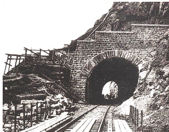
Один из тоннелей на Кругобайкальской железной дороге, 1902 г.
