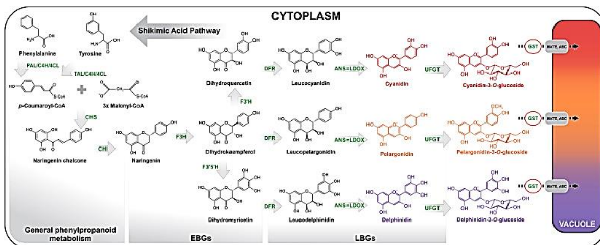
Рис. 13. Схема биосинтеза антоцианов — небольшой фрагмент превращений аминокислоты тирозина в биосфере. По [29]
