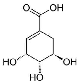
Рис.11. Слева: структурная формула шикимовой кислоты — биохимического предшественника большинства ароматических метаболитов. Справа: плоды бадьяна — природного источника шикимовой кислоты. Изображение с сайта http://3.bp.blogspot.com
