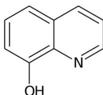
Рис. 3. Слева: 8-гидроксихинолин. Справа: василёк раскидистый. Изображение с сайта https://www.discoverlife.org/
