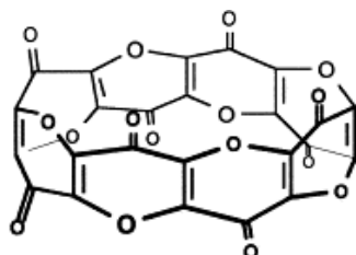
MCS octamer (C 3 O 2 ) 8
