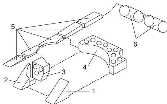
Рис. 2. Система питания топливом танка Т-72: 1, 2 – левый и правый носовые баки; 3, 4 – передний и средний баки-стеллажи; 5 – система наружных топливных баков, расположенных по правому борту; 6 – левая и правая бочки
