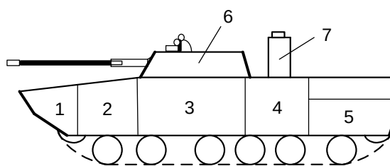
Рис. 1. Машина управления роботанками на базе БМП-3: 1 – отделение носовых топливных баков, выполняющее также роль дополнительной защиты при пробитии брони; 2 – отделение управления, в котором размещается водитель и два оператора роботанков; 3 – боевое отделение; 4 – отделение аппаратуры по управлению роботанками; 5, 6, 7 – соответственно двигательный отсек, башня с вооружением и выдвинутый из бронекорпуса комплекс управления роботанком
