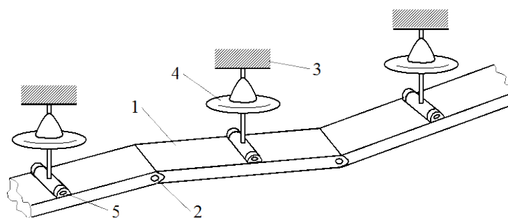
Рис. 6. Токопровод с боковой рабочей поверхностью
