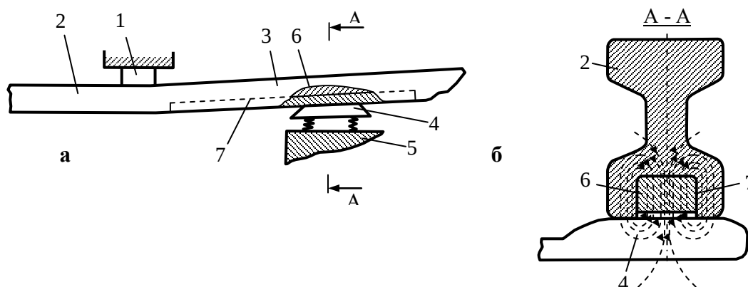
Рис. 8. Схема концевой отвода, разработанного в ОмГУПСе:
