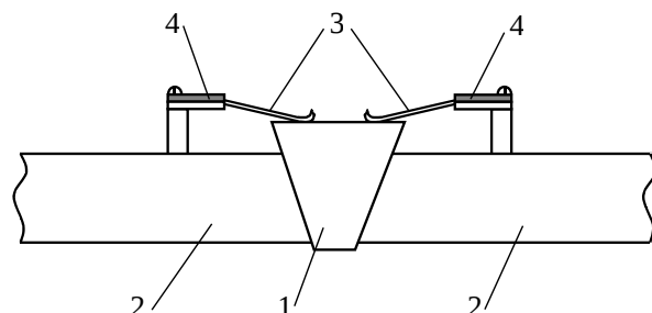
Рис. 7. Стыковой соединитель жесткого токопровода
