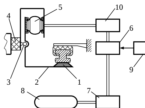
Рис. 4. Токоприемник ТР-3м
