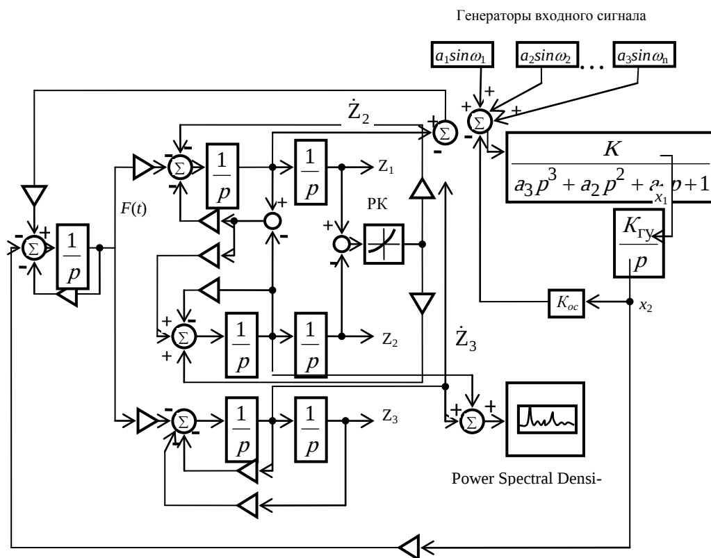
Рис. 4. Схема моделирования в среде Matlab с расширением Simulink
