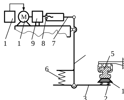
Рис. 5. Токоприемник ТРЭП
