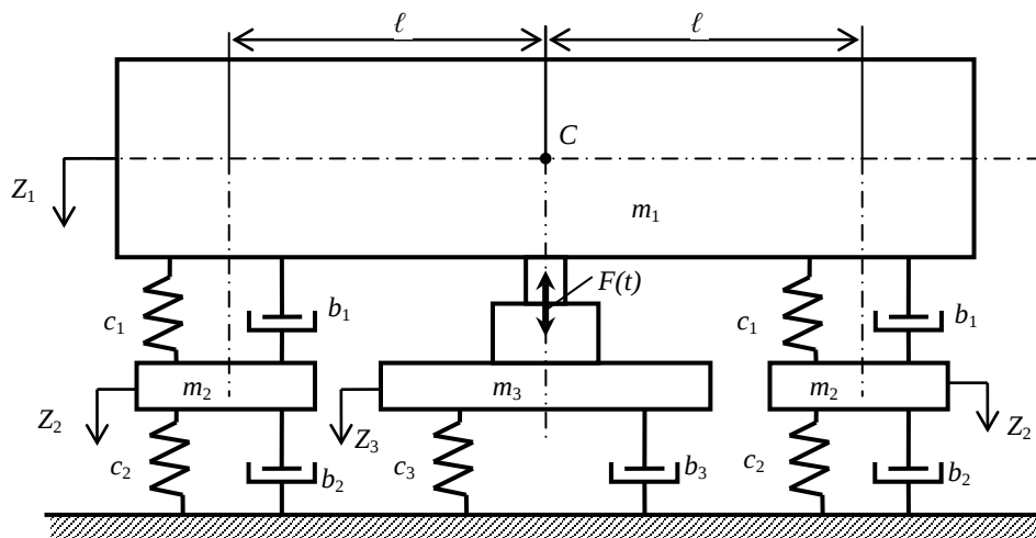
Рис. 2. Схема расчётная:
