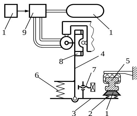
Рис. 3. Токоприемник ТРКП
